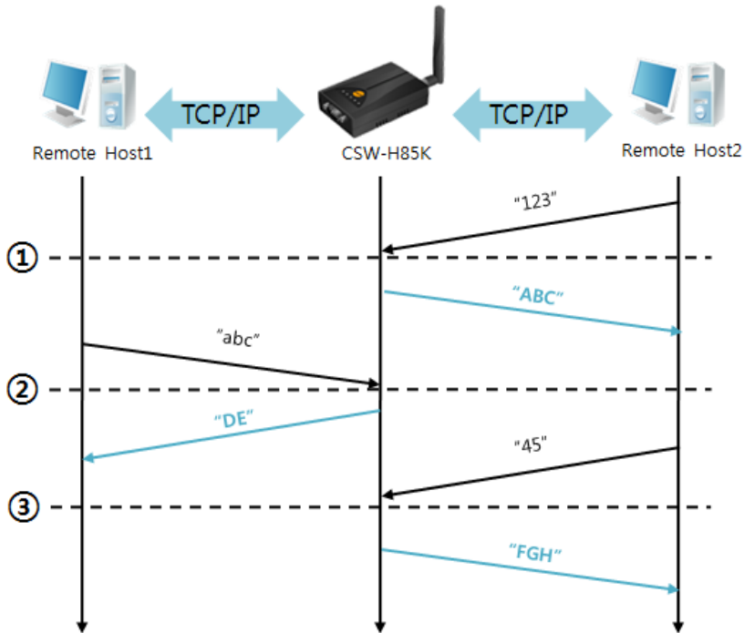
图 5-11 UDP动态HOST传送例
