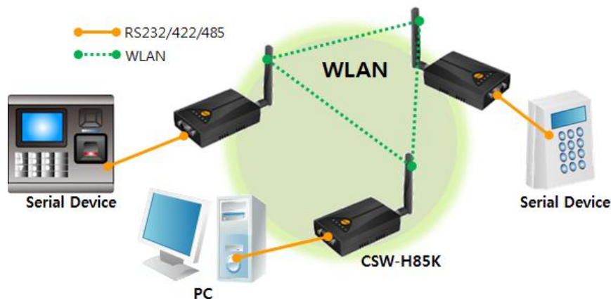
图2-3 Ad-hoc
