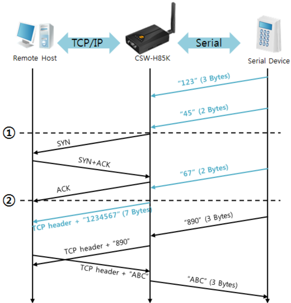
图 5-5 连接前数据大小为5的情况
