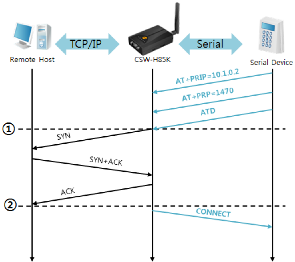
图 5-8 TCP 自动连接
