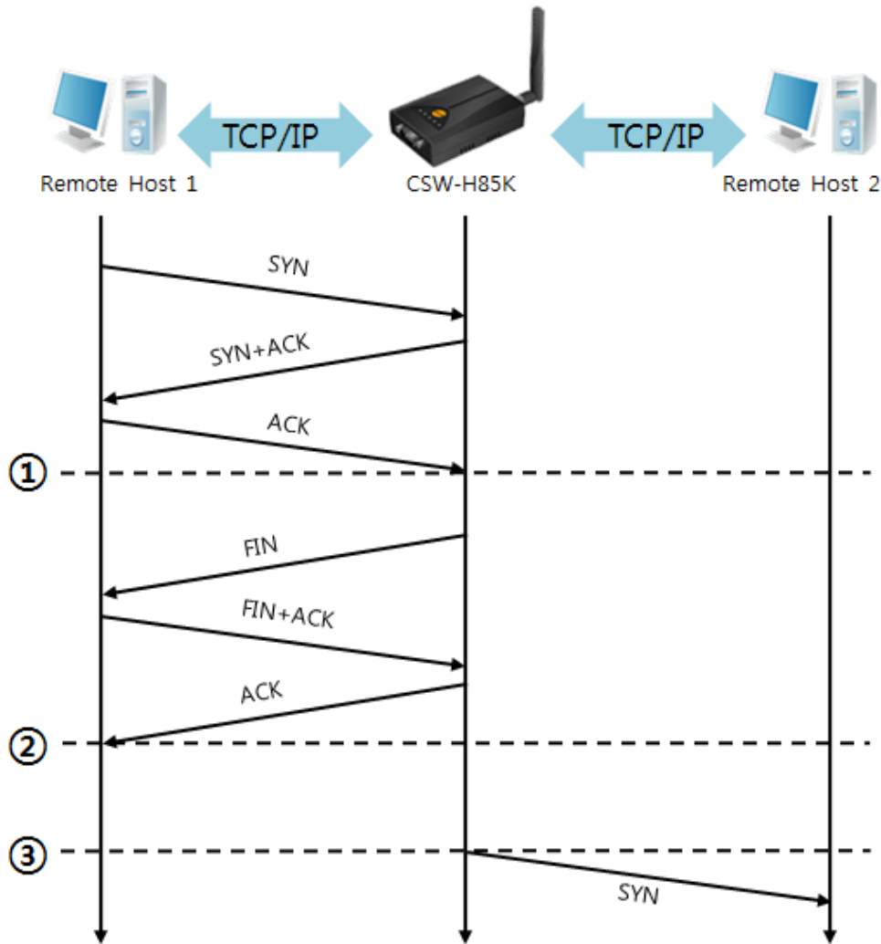
图 5-6 TCP 服务器/客户端模式时
