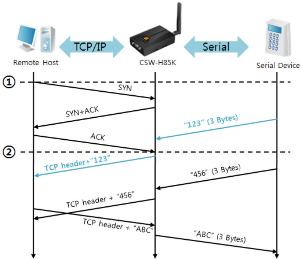
图 5-2 连接前数据大小为1的情况
