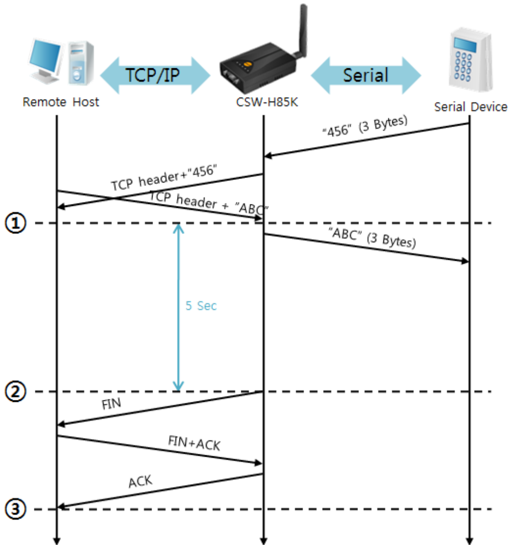
图 5-3等待时间为5的情况
