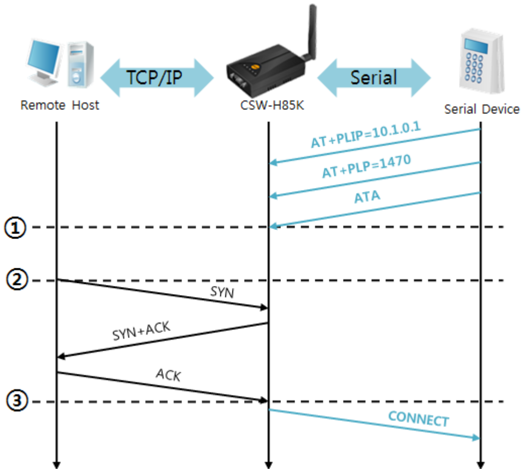
图 5-7 TCP 手动连接
