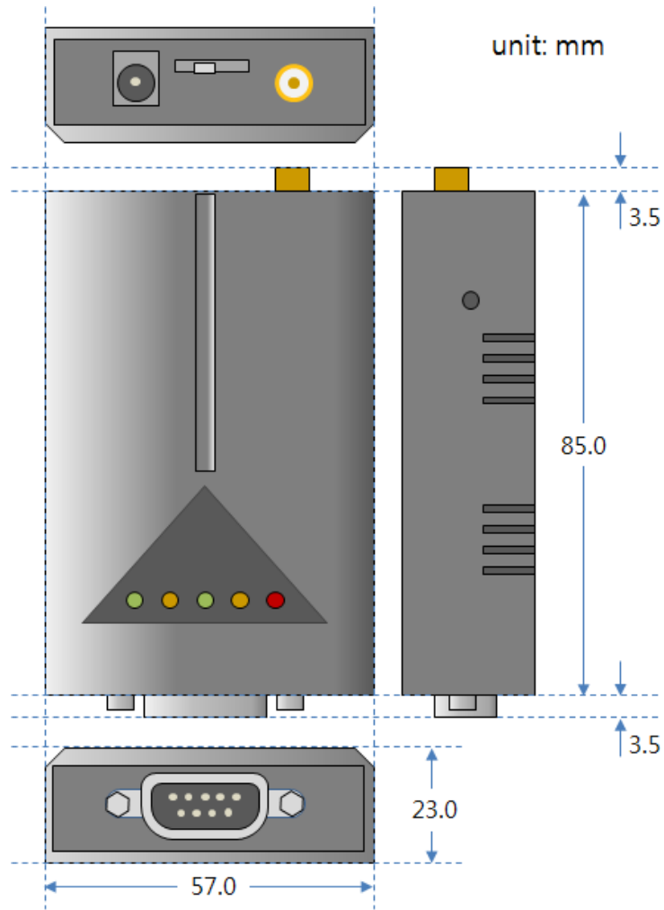
图 1-4 CSW-H85K尺寸
