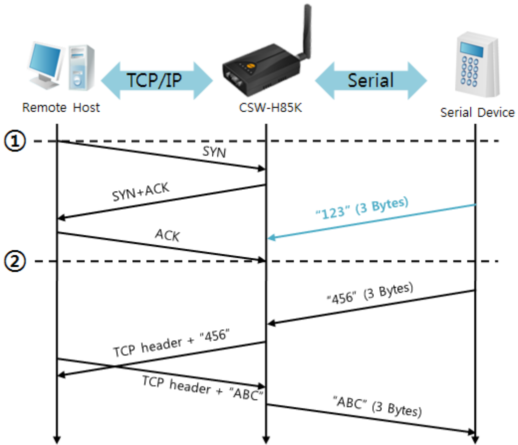
图 5-1 连接前数据代谢大小为0的情况
