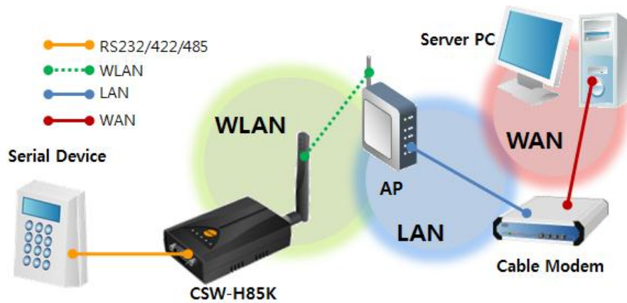
图 1-3 利用xDSL/电缆调制解调器的因特网连接
