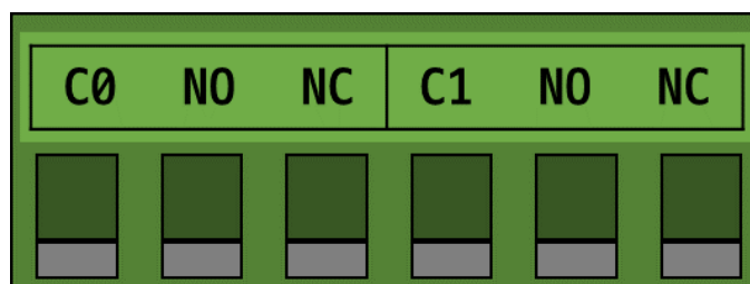
Схема 1-4 Порт цифрового вывода
