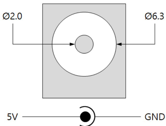
Схема 1-2 Питание
