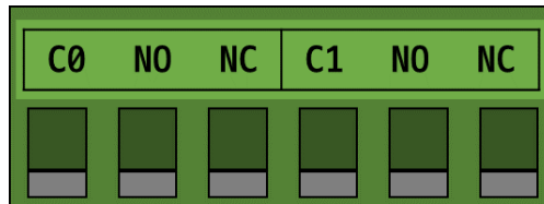
그림 1-4 디지털 출력 포트
