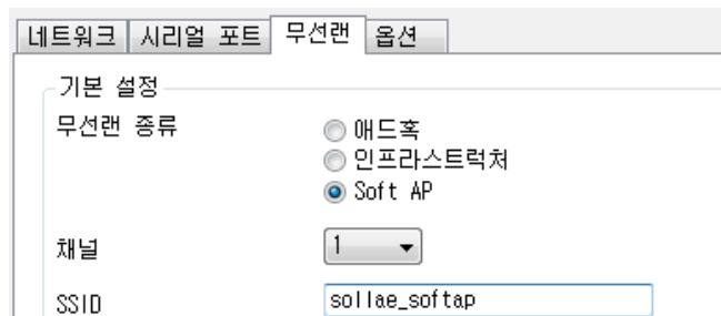
그림 2-6 Soft AP 모드 설정
