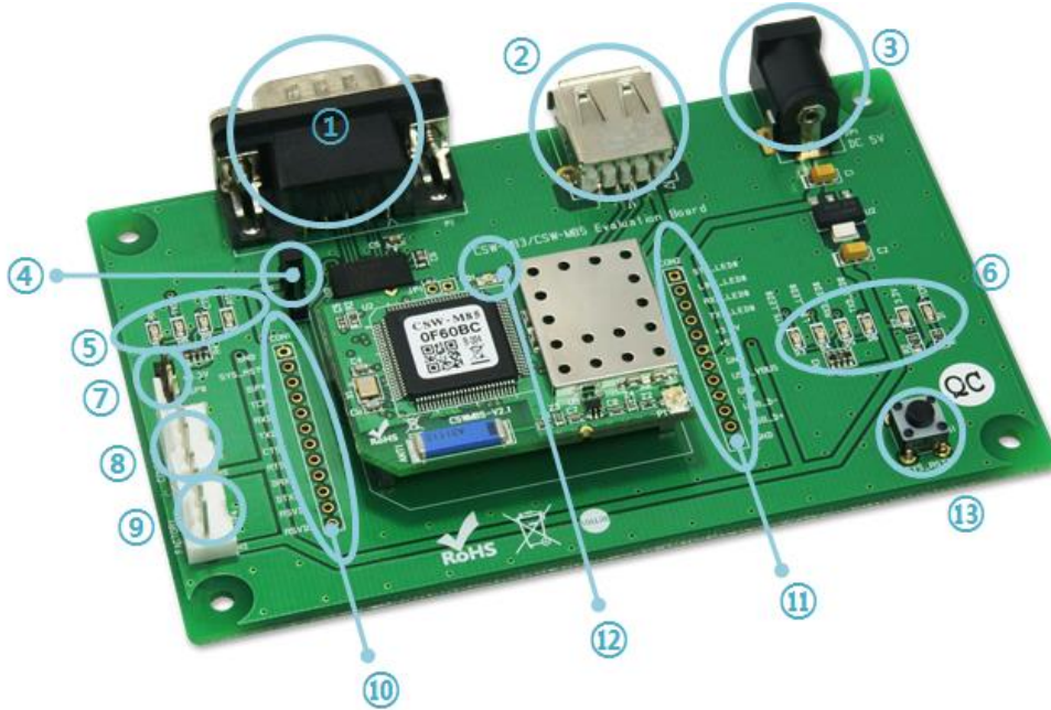
그림 1-7 개발용 보드
