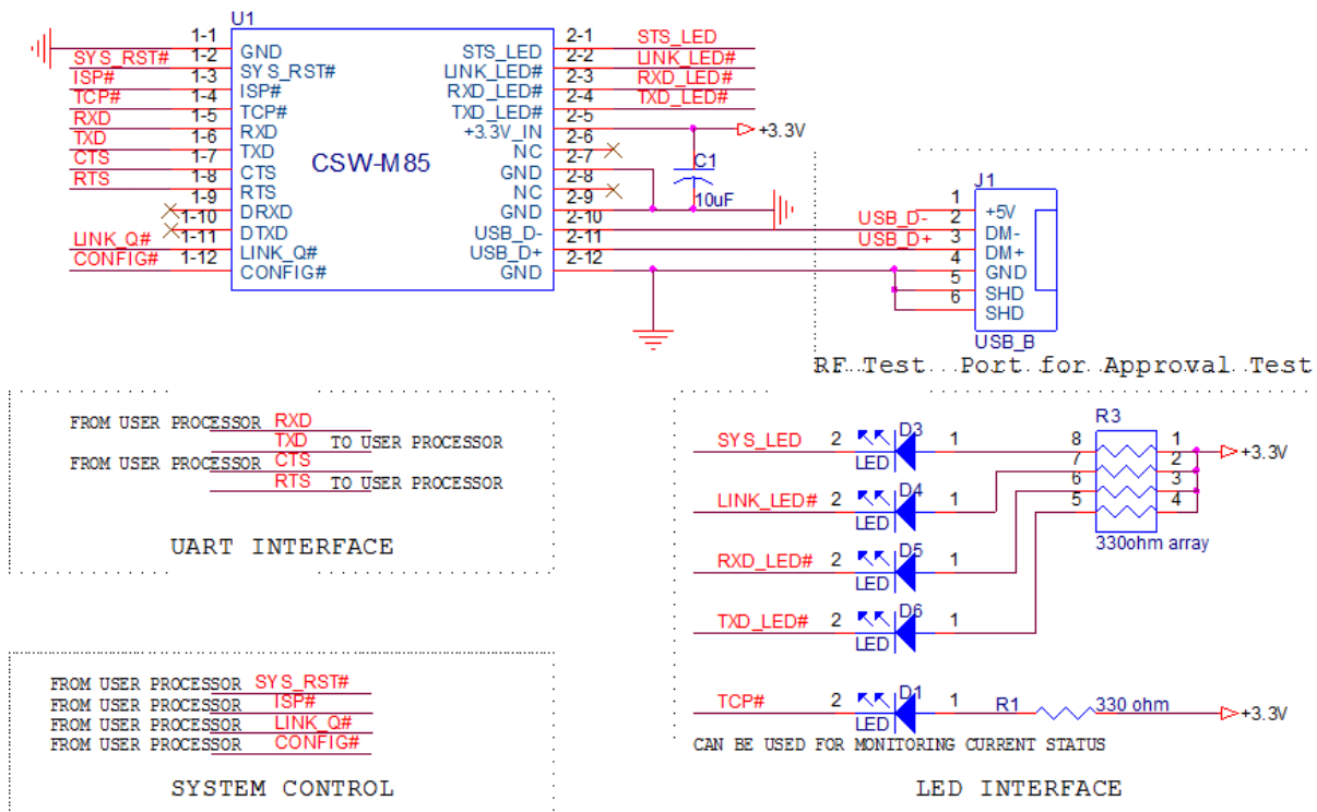
그림 1-6 응용 회로도
