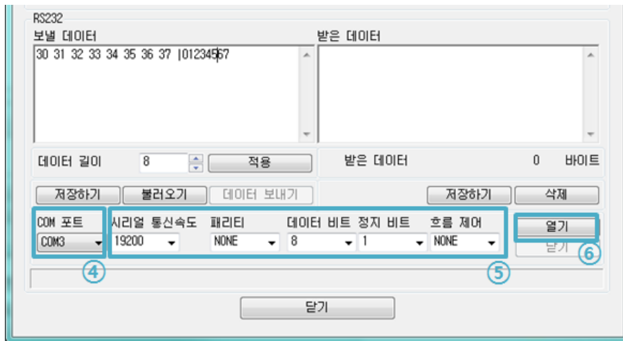
그림 2-15 시리얼로 COM 포트 열기
