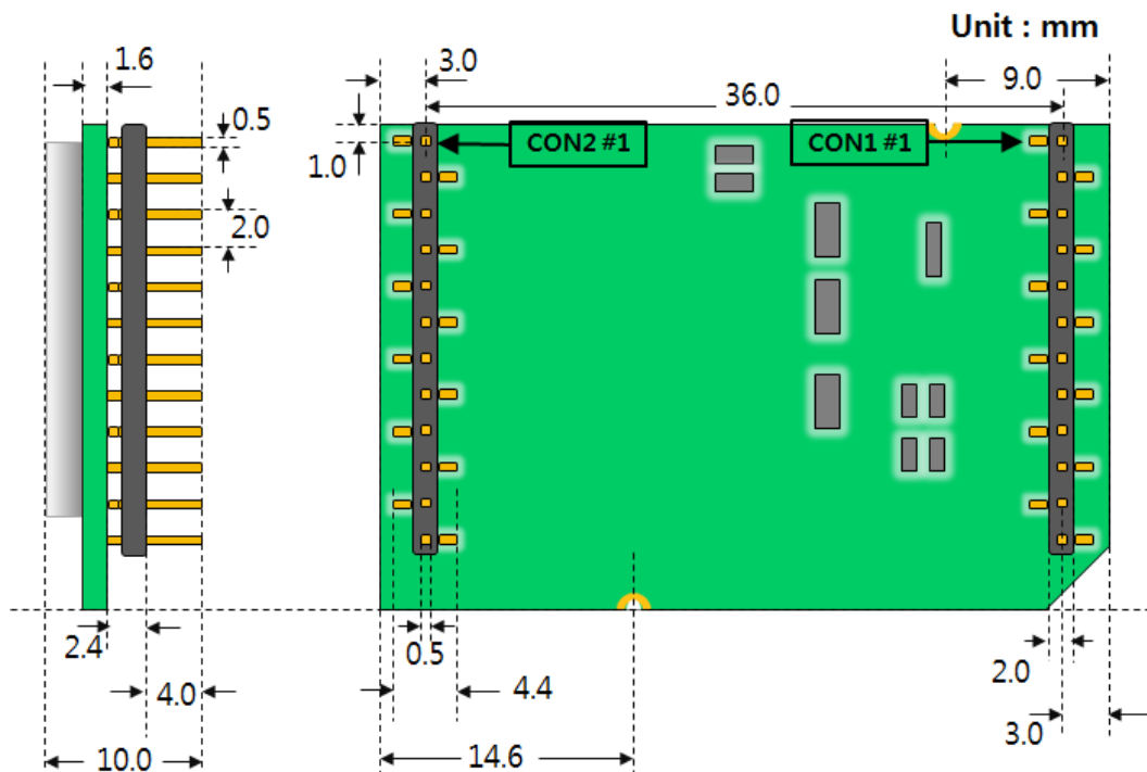
그림 1-5 Side / Bottom view
