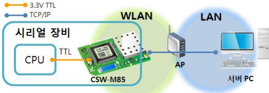
그림 1-2 AP를 이용한 내부 네트워크 연결
