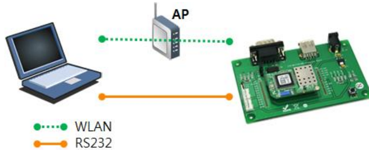
그림 2-7 노트북을 이용한 시험작동 시 구성
