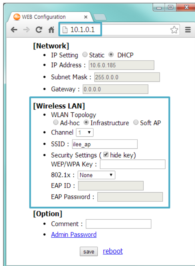
그림 2-11 웹 설정 페이지 접속
