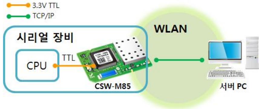
그림 1-1 무선랜 연결 가능한 PC와 1:1 연결
