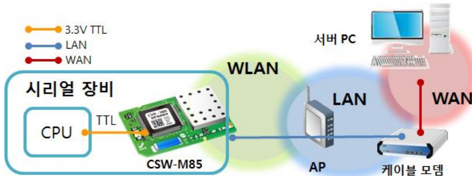
그림 1-3 xDSL/케이블 모뎀을 이용한 인터넷 연결
