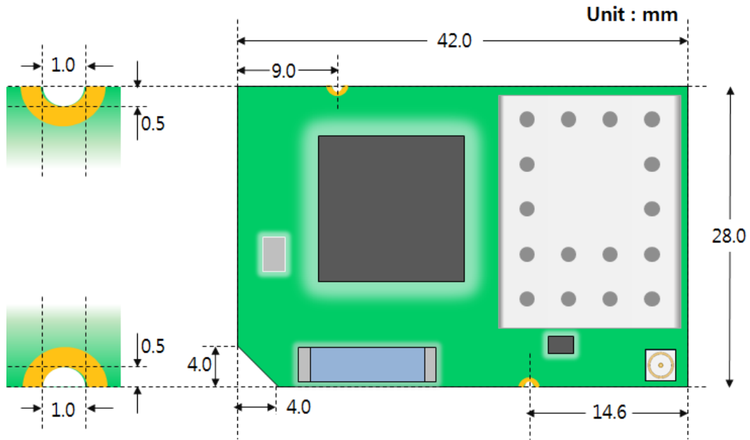
그림 1-4 Top view
