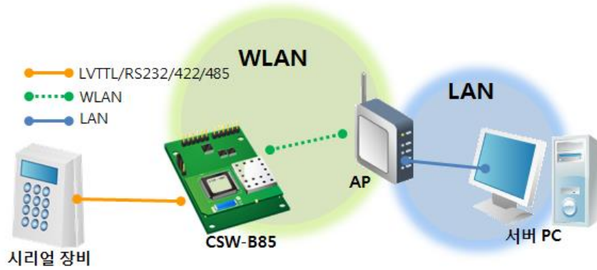
그림 1-2 AP를 이용한 내부 네트워크 연결
