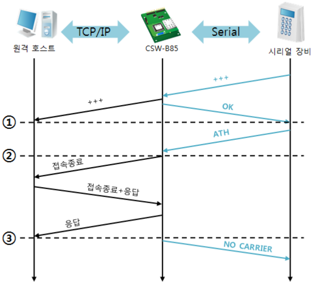
그림 5-9 TCP 접속종료
