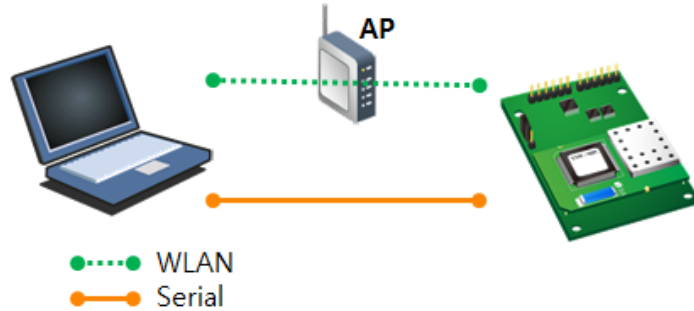
그림 2-7 노트북을 이용한 시험작동 시 구성
