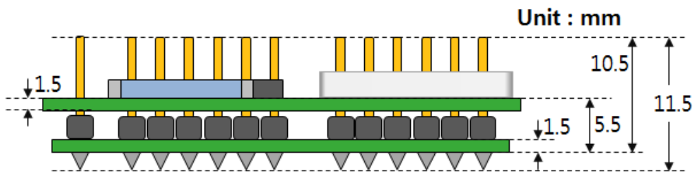
그림 1-5 Side view
