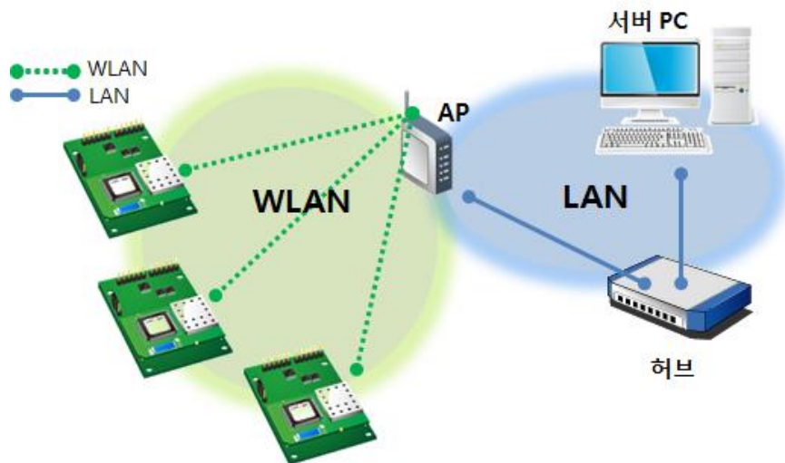
그림 2-1 인프라스트럭처 모드
