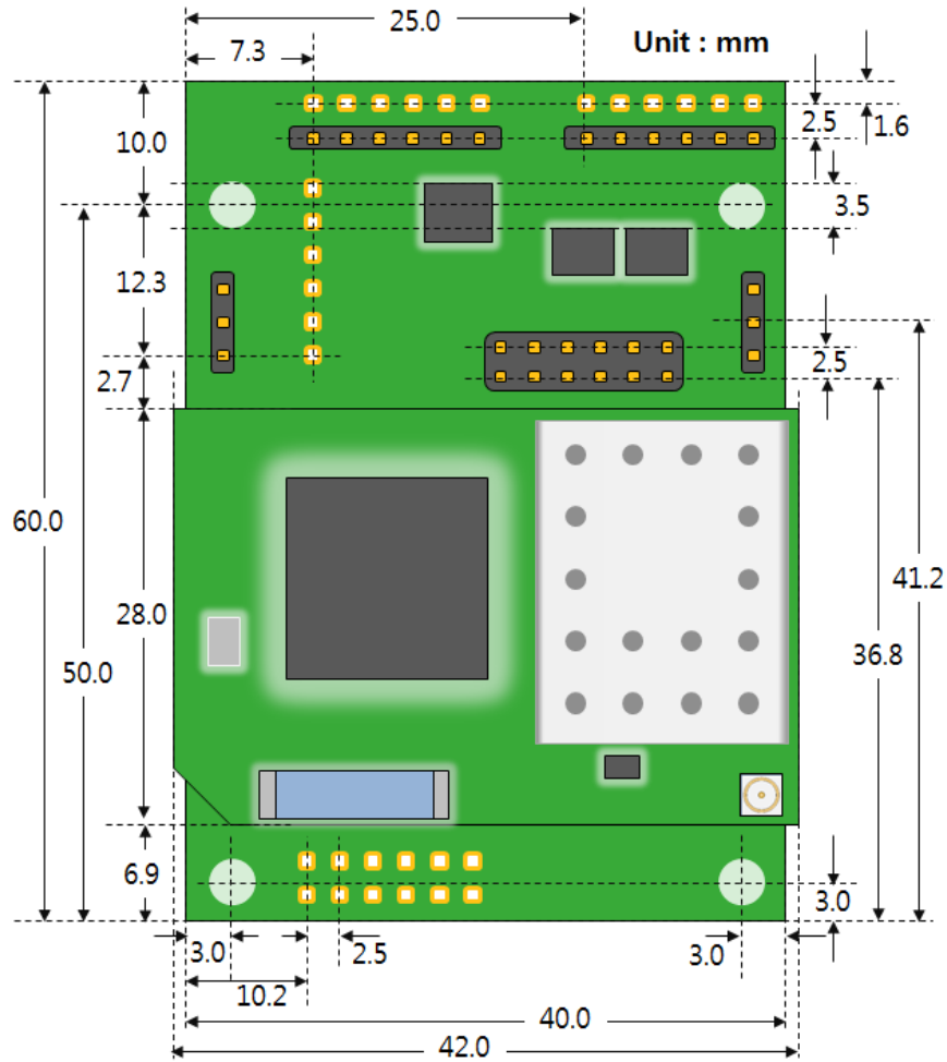
그림 1-4 Top view
