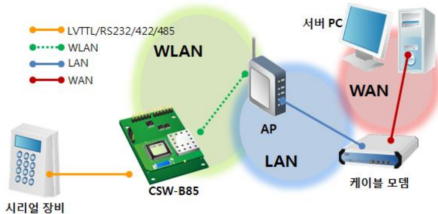
그림 1-3 xDSL/케이블 모뎀을 이용한 인터넷 연결
