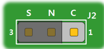
그림 7-8 수신신호강도표시기능 설정
