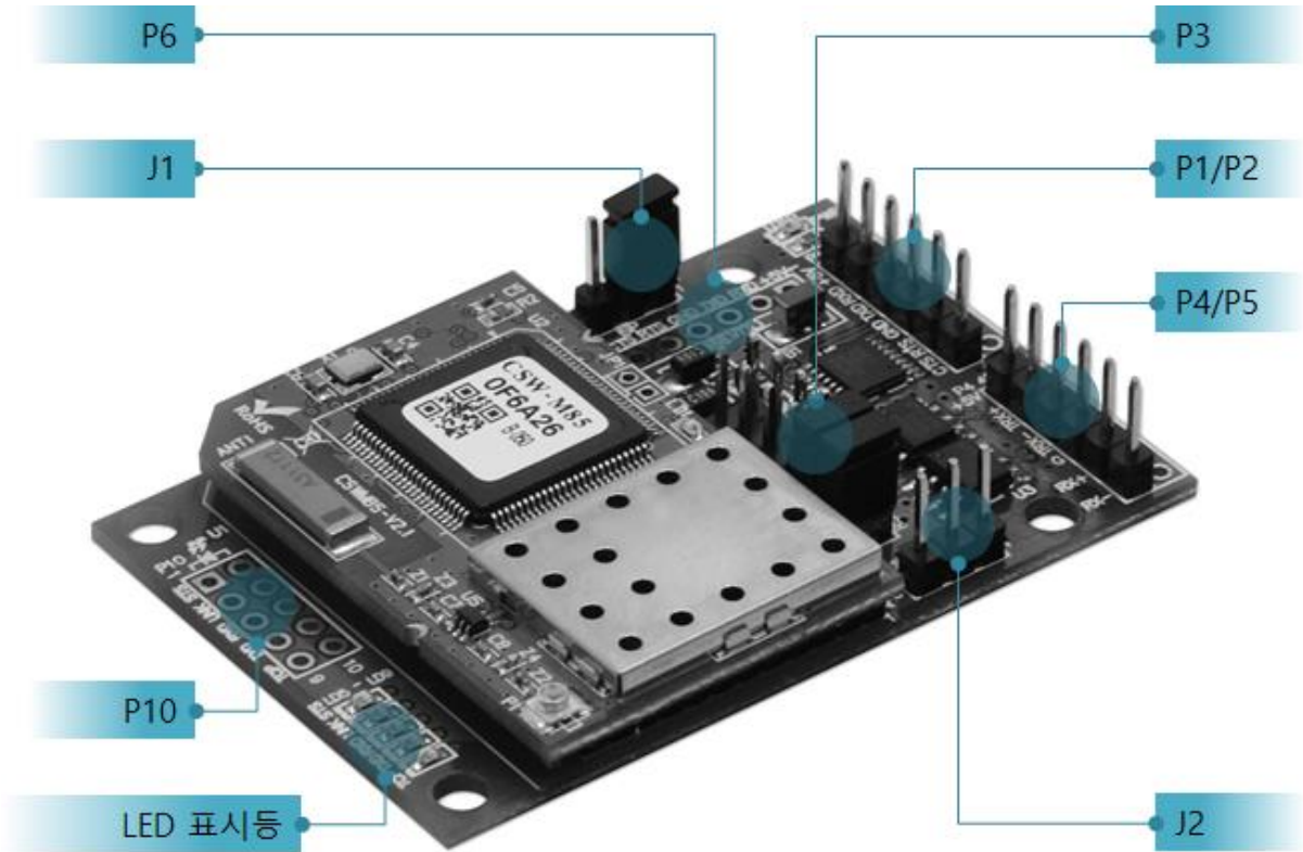
그림 1-6 인터페이스
