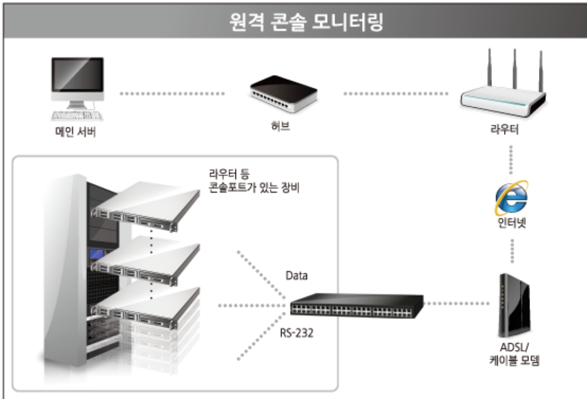
그림 1-1 CSE-T48 구성도
