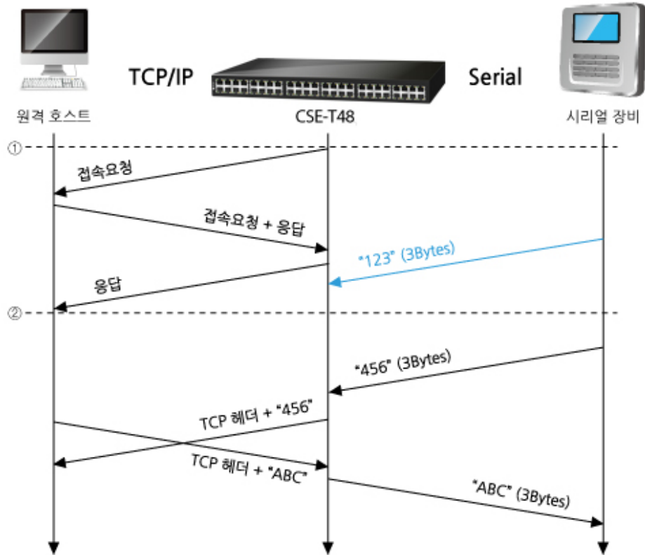
그림 4-3 접속 전 데이터 크기가 0인 경우
