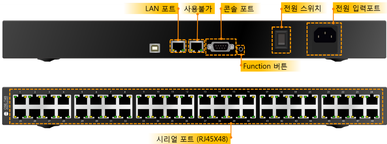
그림 1-3 CSE-T48 패널 레이아웃
