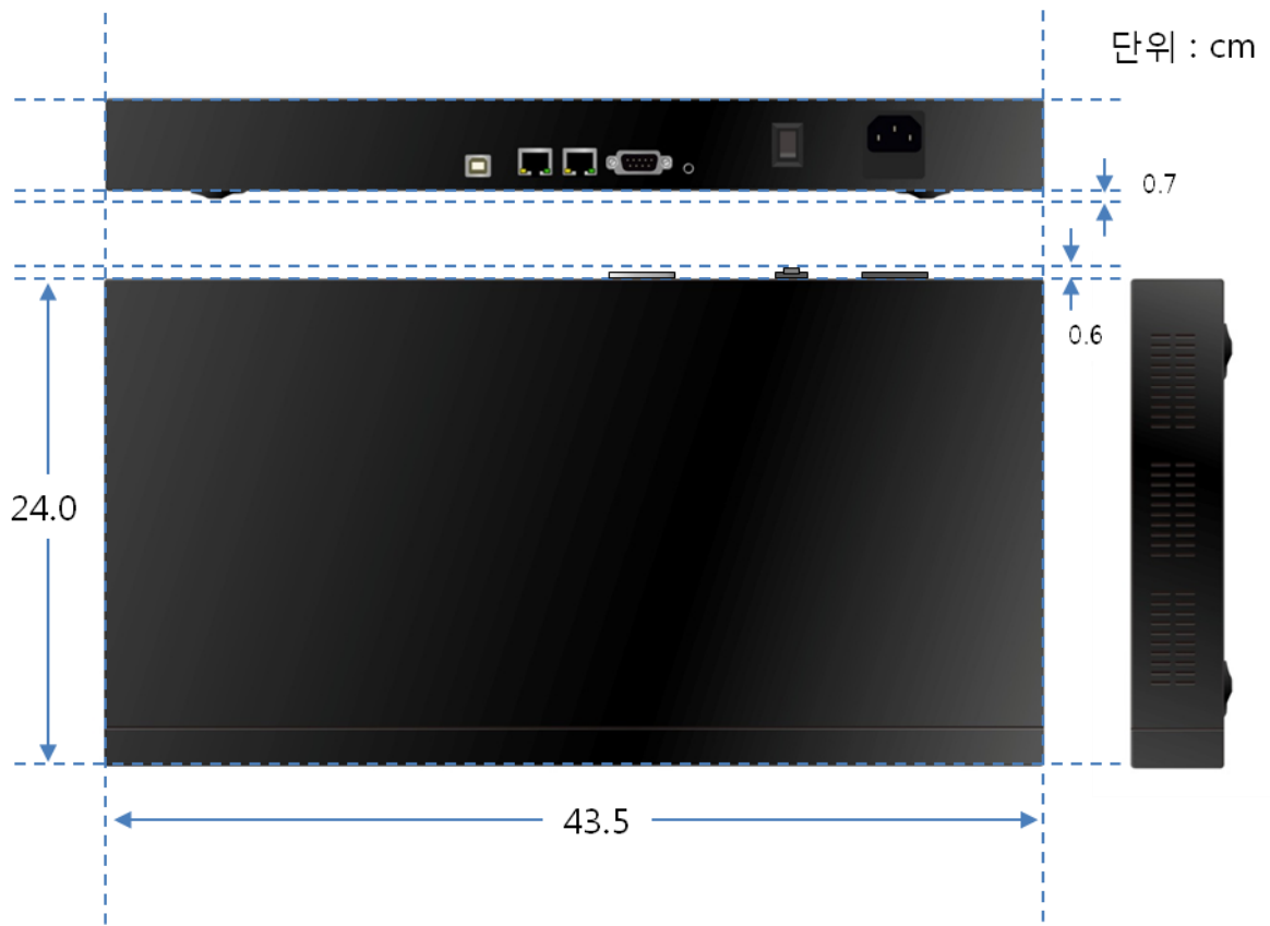
그림 1-2 치수
