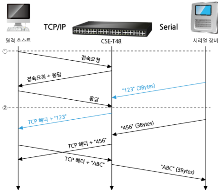
그림 4-2 접속 전 데이터 크기가 1인 경우
