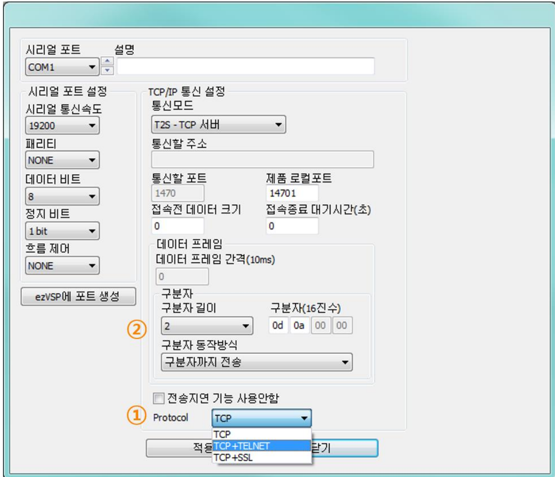
그림 7-1 CSE-T48 탭 기능
