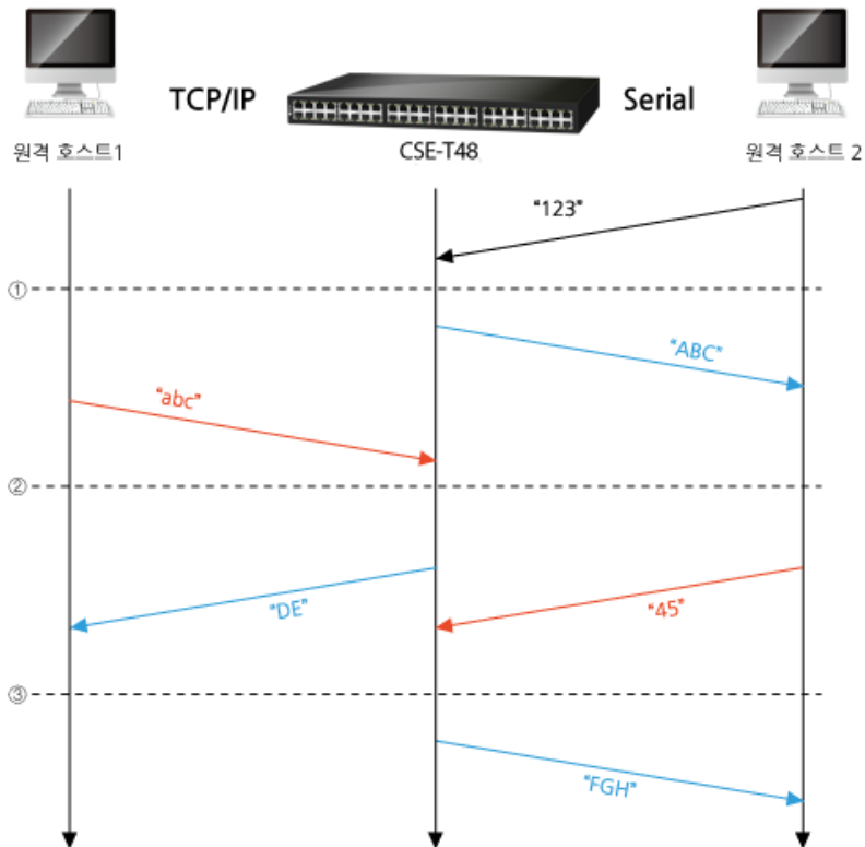
그림 4-6 UDP 동적 호스트 전송 예
