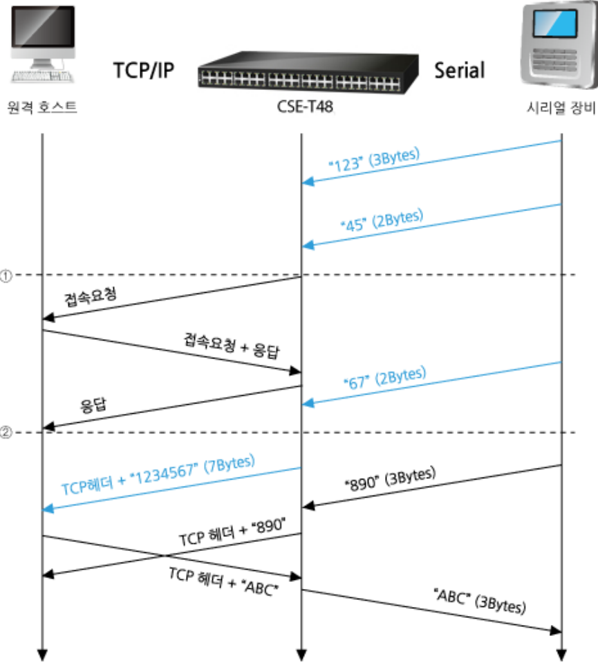
그림 4-4 접속 전 데이터 크기가 5인 경우
