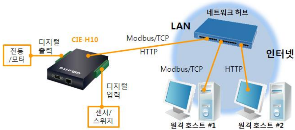
그림 1-1 원격 디지털 입/출력 감시/제어 구성 예
