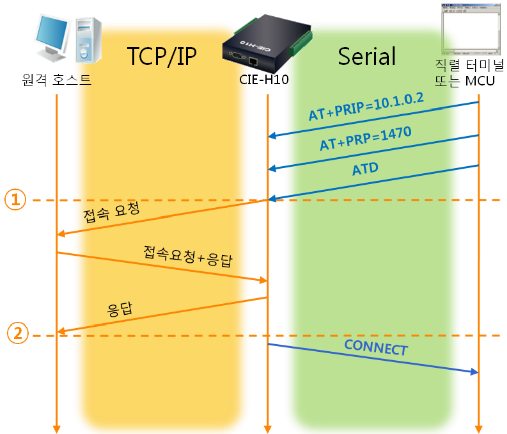
그림 6-5 TCP 능동접속
