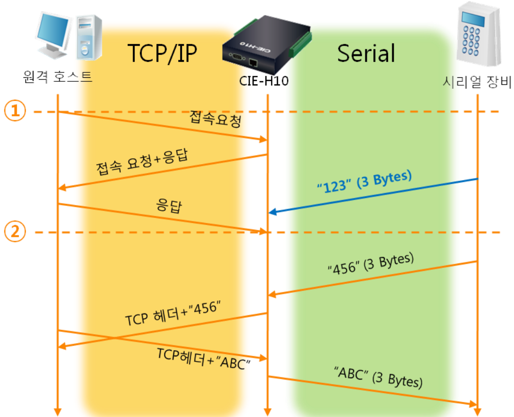
그림 6-1 TCP 서버
