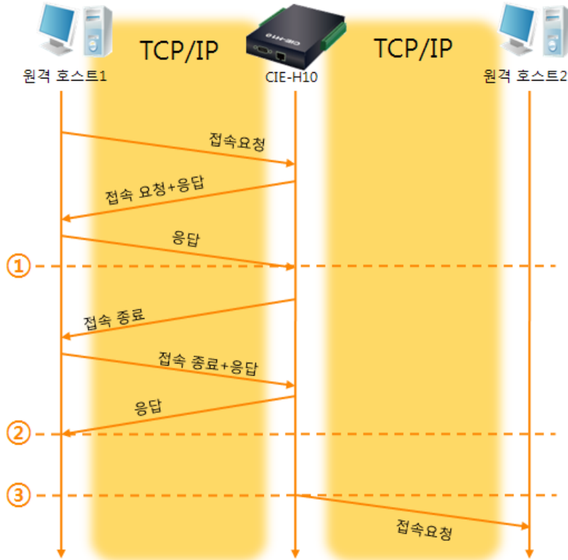
그림 6-3 TCP 서버/클라이언트
