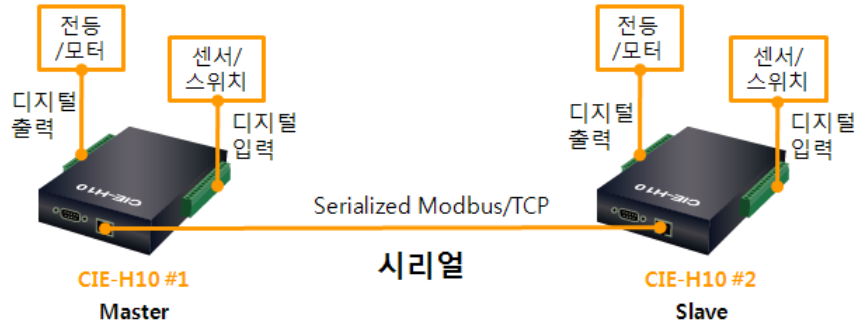
그림 1-4 시리얼 스위치 구성 예
