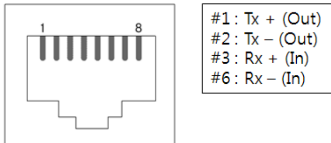
그림 1-10 RJ45 이더넷 커넥터 사양
